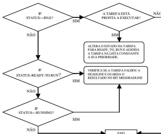
Fig. 3 - Função Tick() - (em EDF a prioridade instantânea é indicada no campo Aux do TCB)
