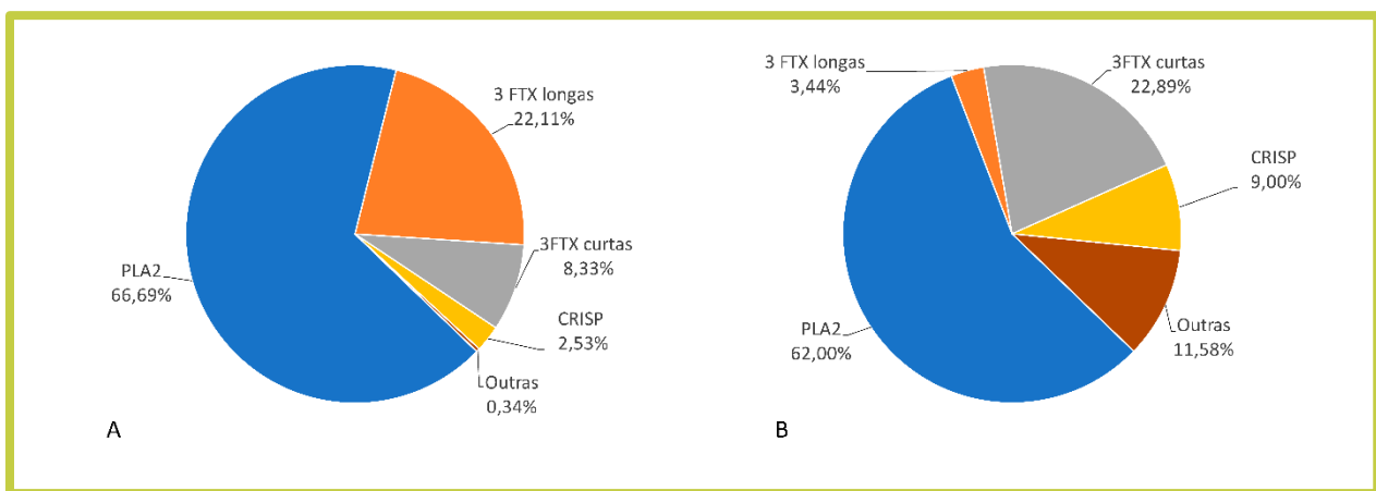
FIGURA 1: Variabilidade intraespecífica no proteoma de Hydrophis curtus . A – Indivíduos capturados na Austrália. B – Indivíduos capturados na Malásia. PLA2 – Fosfolipase A2; 3FTX – Three finger toxins; CRISP - Cysteine-rich secreted proteins.
